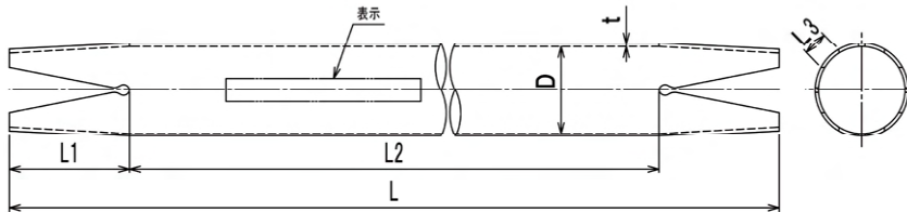
A型（筒形状）
