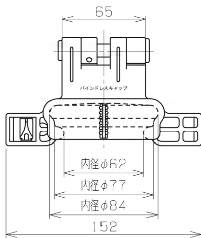
〔ツメ形状固定タイプ〕
