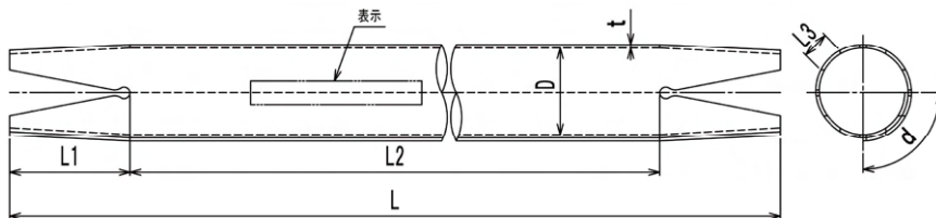
B型（半割形状）
