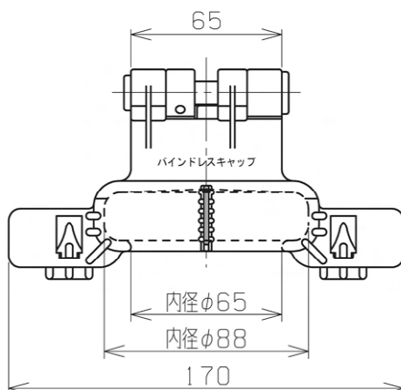
〔ツメ形状脱着タイプ〕
