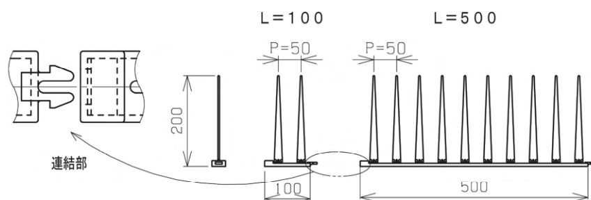
アーム用飛来防止器 連結タイプ
